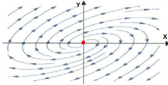
Figura 7.12: Punto espiral inestable
