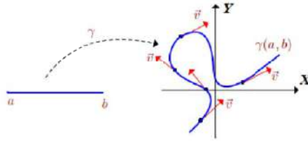
Figura 7.1: Trayectoria de una partícula en el plano
