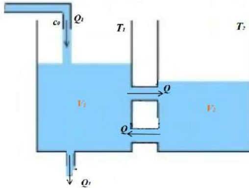
Figura 6.1: Sistemas de tanque conectados.
