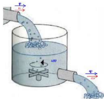
Figura 2.1: Mezcla de sustancias en un tanque.
