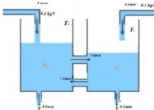
Figura 6.2: Sistema de tanques conectados T_1 y T_2 .
