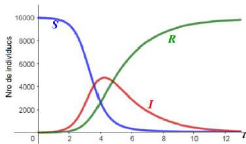
Figura 7.13: Modelo SIR caso epidemiológico
