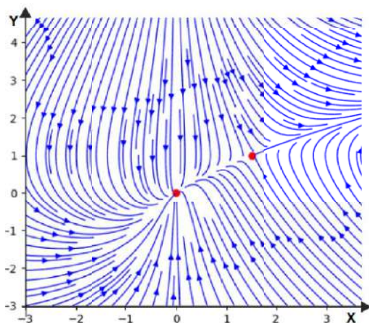
Figura 7.16: Diagrama fase del sistema \begin{cases} x' = xy - x \\ y' = 2x - 3y \end{cases} .
