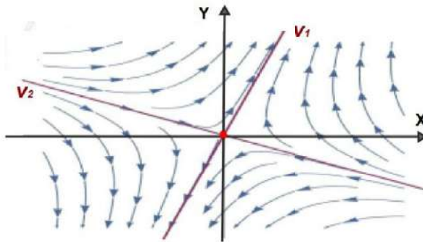
Figura 7.5: Punto silla
