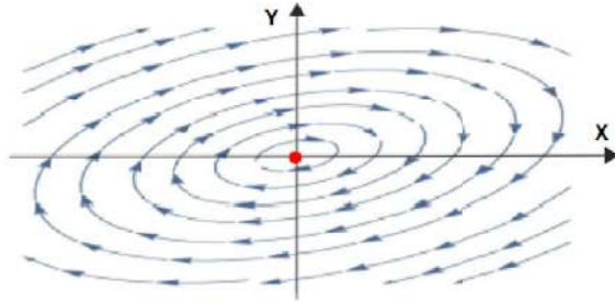
Figura 7.10: Punto centro estable
