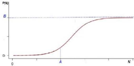
Figura 2.4: Función P(N) no lineal.
