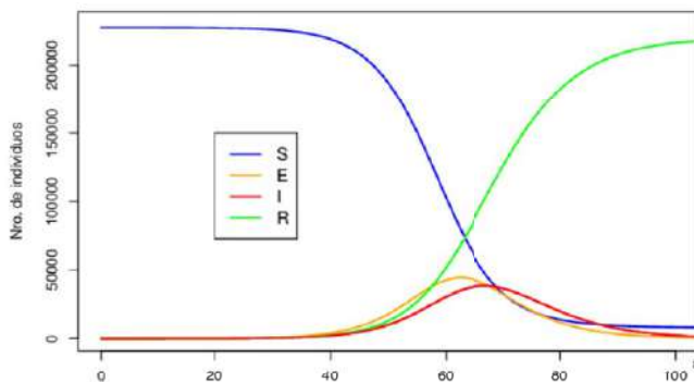
Figura 7.14: Modelo SEIR caso epidemiológico
