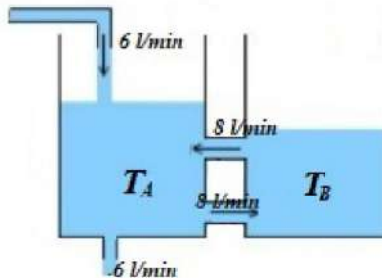
Figura 6.3: Sistema de tanques conectados T_A y T_B .
