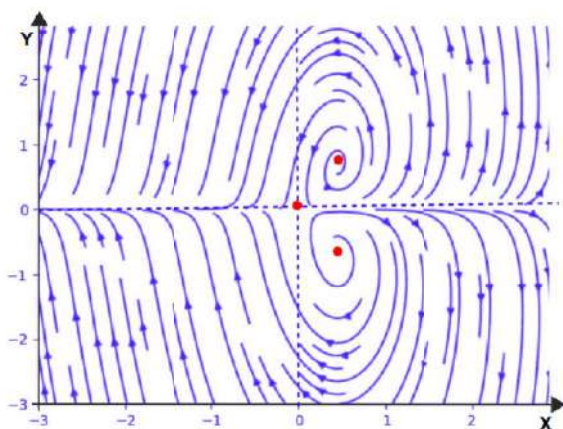
Figura 7.17: Diagrama de fase del sistema \begin{cases} x' = x - y^2 \\ y' = y(9x - 4) \end{cases}
