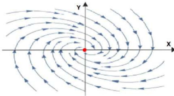
Figura 7.11: Punto espiral estable
