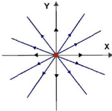
Figura 7.7: Nodo inestable un autovalor positivo y dos autovectores l.i.
