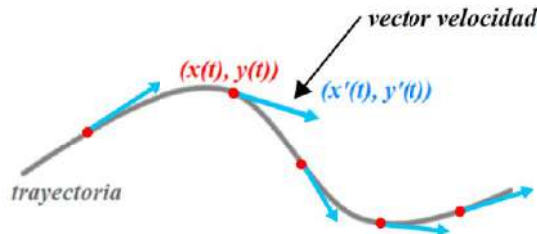
Figura 7.2: Vectores tangentes a una trayectoria
