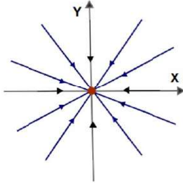
Figura 7.6: Nodo estable un autovalor negativo y dos autovectores l.i.
