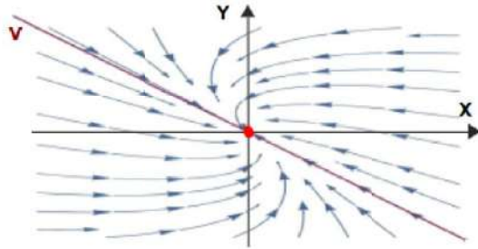
Figura 7.8: Nodo impropio estable
