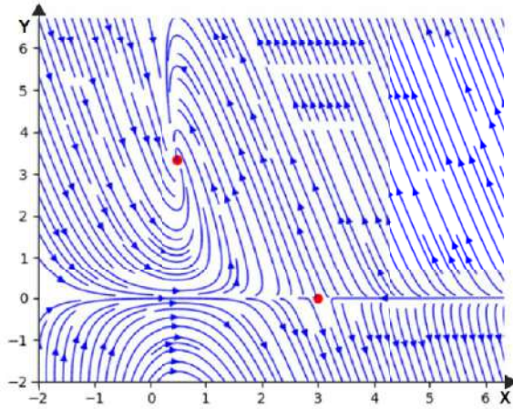
Figura 7.15: Diagrama de fase del sistema \begin{aligned} x' &= 2\left(1 - \frac{x}{3}\right) - xy \\ y' &= -2y + 4xy \end{aligned}
