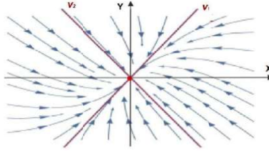
Figura 7.3: Nodo estable
