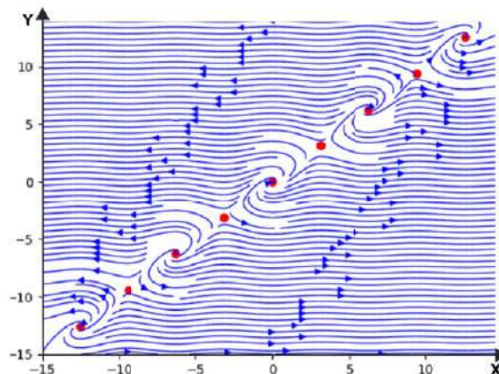
Figura 7.18: Diagrama de fase del sistema \begin{cases} x' = x - y \\ y' = \sin x \end{cases}
